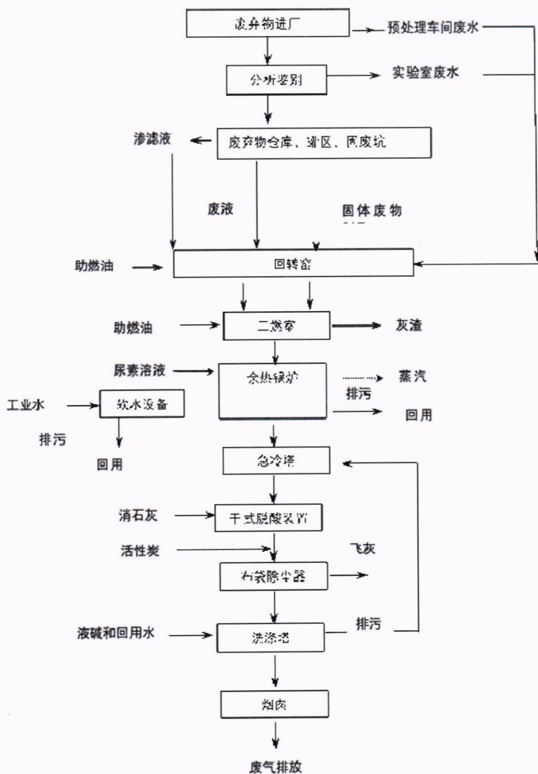
工艺流程及产污环节图
