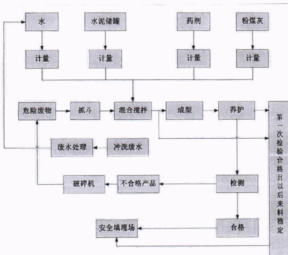
图 2-1 固化/稳定化工艺流程图
