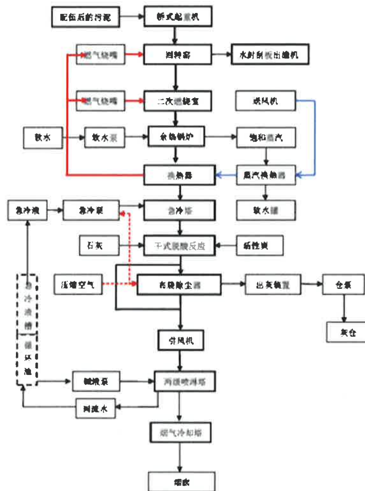
图 4-1 本项目污泥烧结工艺流程图
