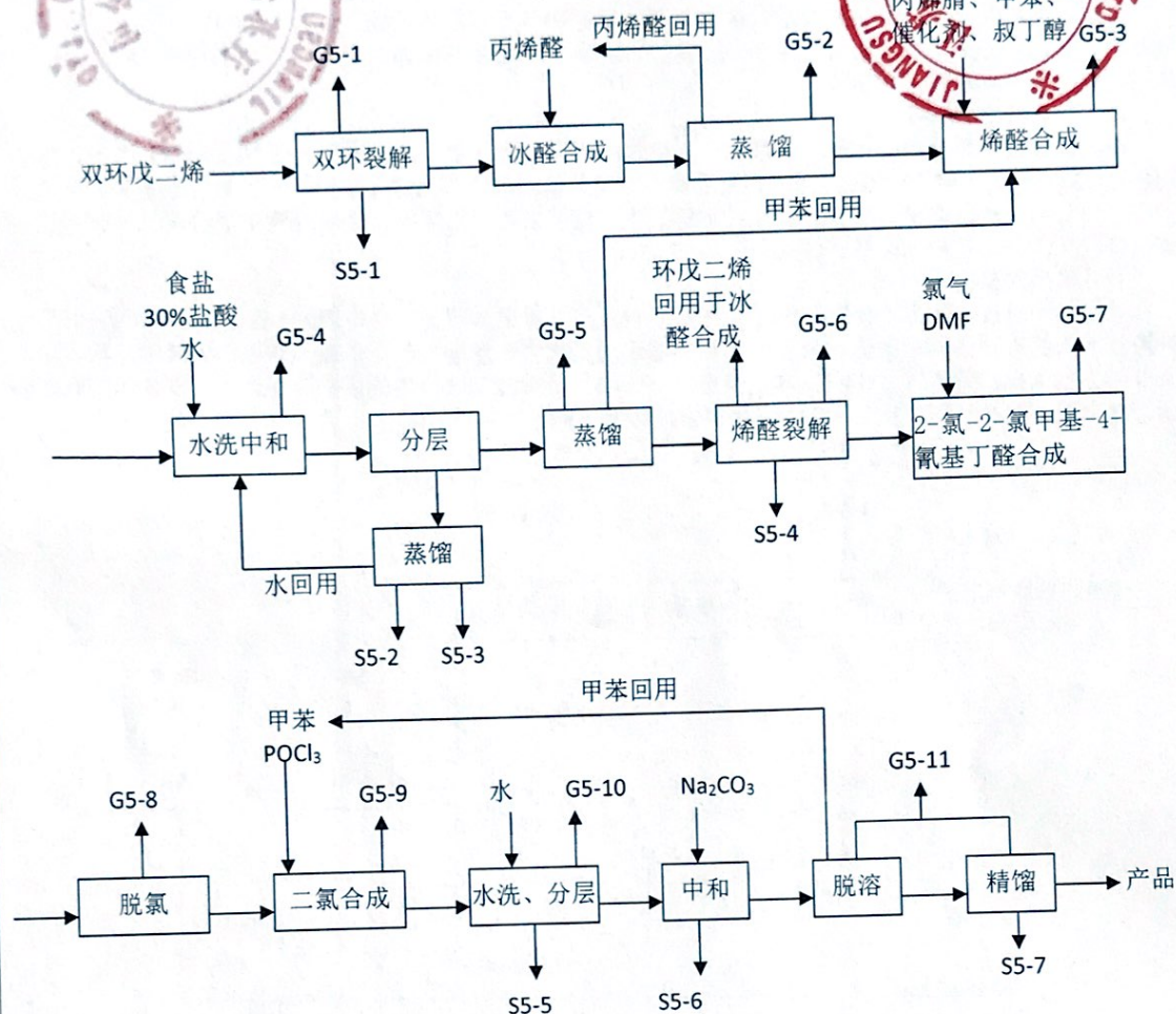
2-氯-5-氯甲基吡啶生产工艺流程图
