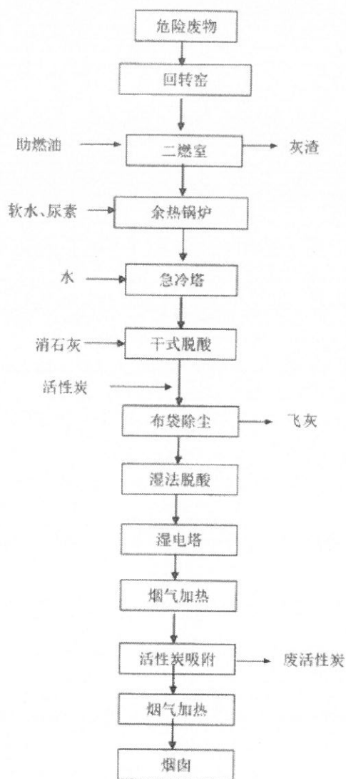
危险废物焚烧处置工艺流程图
