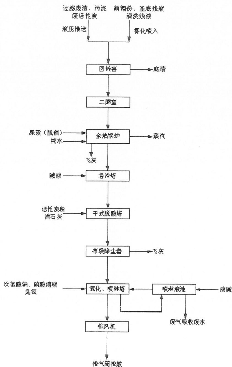
图3-3-3-1 本项目焚烧系统工作流程示意图
