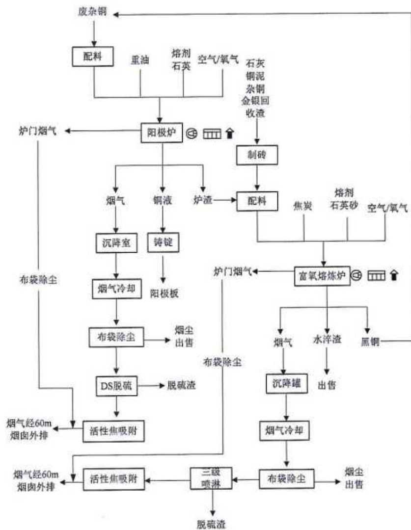
富氧熔炼炉工艺流程见图
