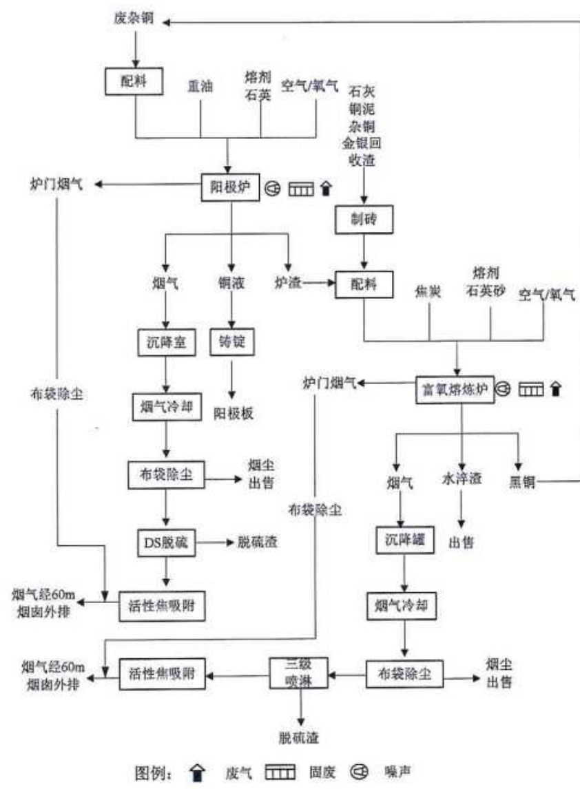
阳极炉工艺流程见图
