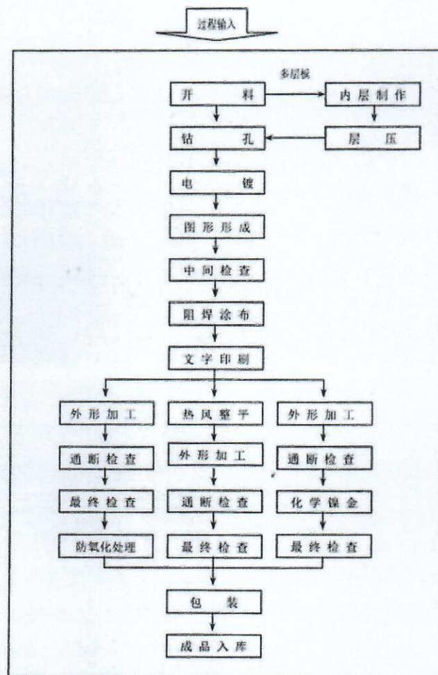
制造工艺流程图
